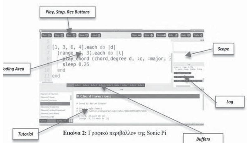
Εικόνα 2 Γραφικό περιβάλλον της Sonic Pi
