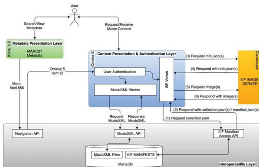
Αρχιτεκτονική Αποθετηρίου
